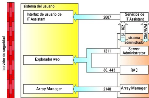
Figura 11-1. Instalación típica detrás de un servidor de seguridad
