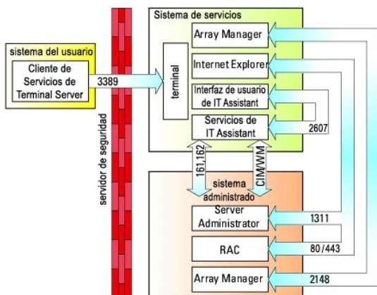
Figura 11-2. Cómo utilizar los servicios de Terminal Server para obtener seguridad adicional
